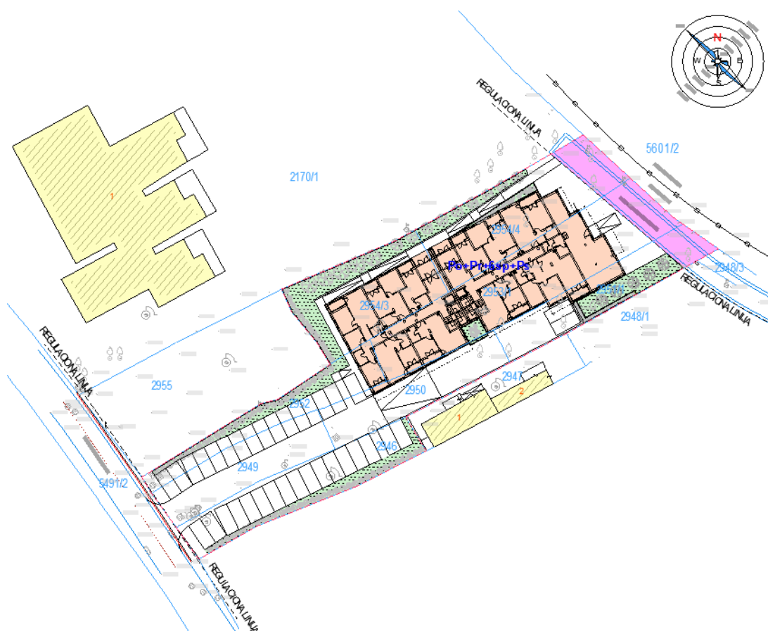
sl. 04 - Situacioni prikaz dispozicije objekta u obuhvatu UP
